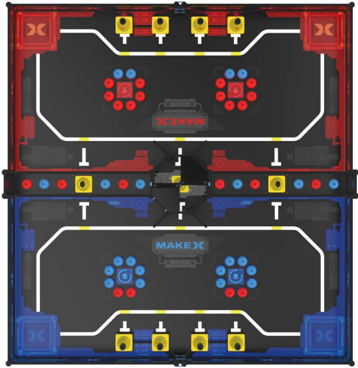
图 4.2-2 场地俯视图
