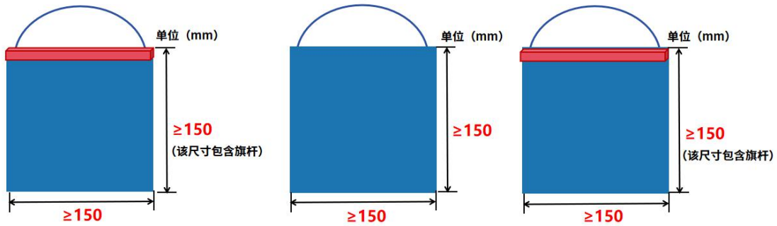
图 4.3-3 净网旗帜示意图
